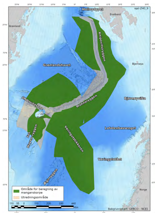
Fig. 6.2 Område for ressursberegning for manganskorper
