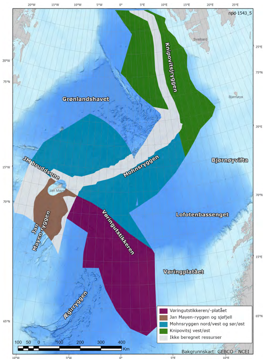
Fig. 4.28 Regionale områder for beregning av manganskorper
