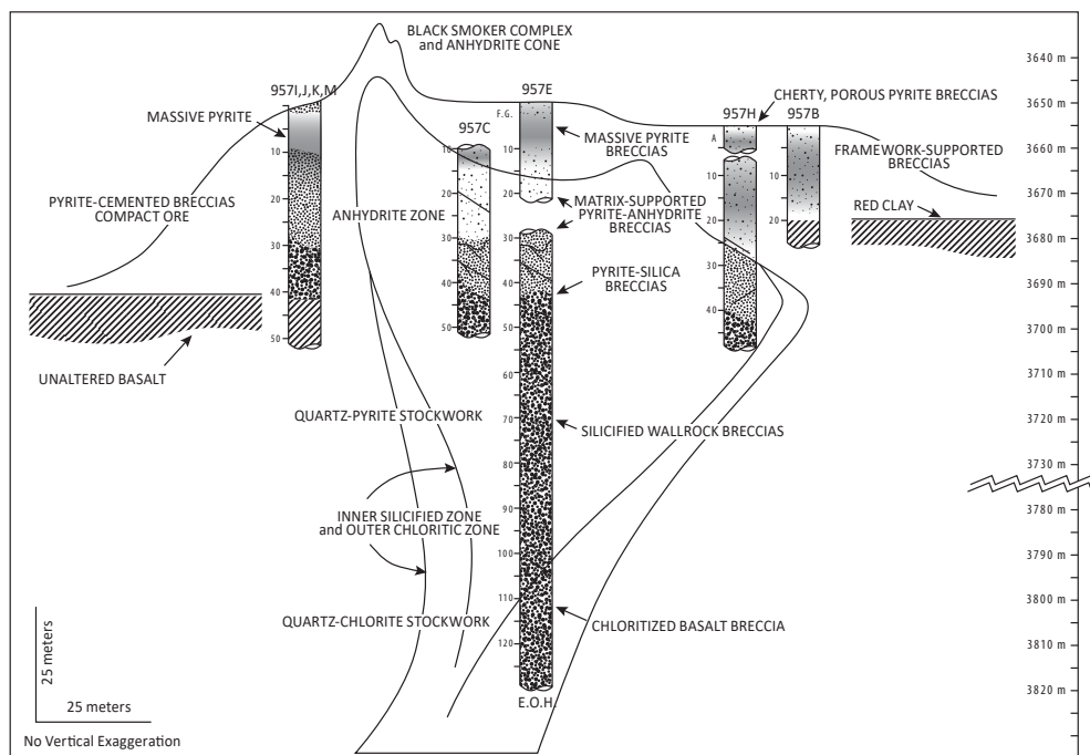
Fig. 4.11 TAG sulfidforekomst
